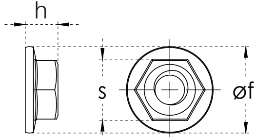
Flange Nut
