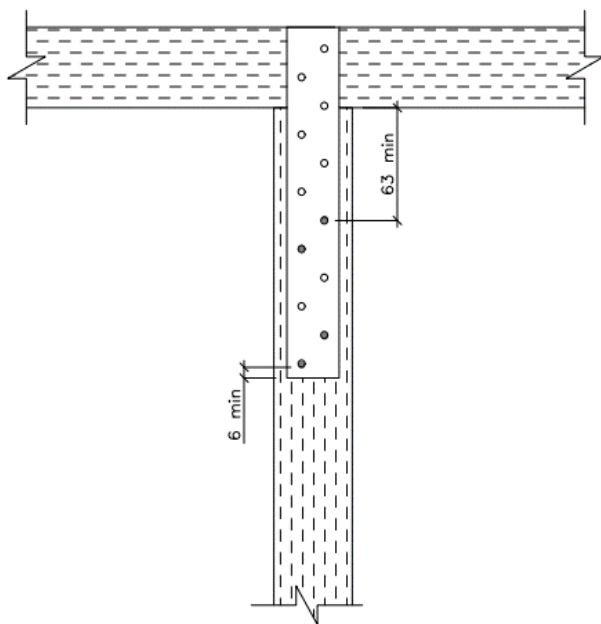
Figure N.1 Minimum Edge and End Distances.
